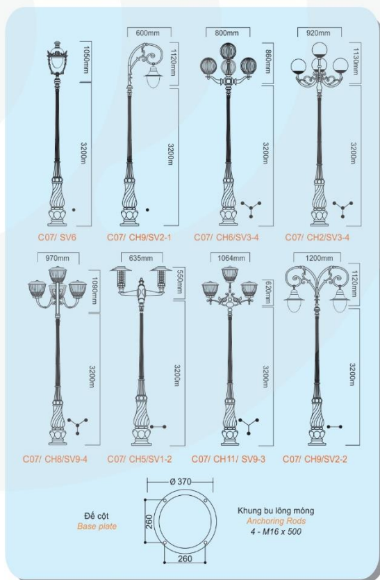
CỘT ĐÈN TRANG TRÍ ĐẾ GANG C07 | C07 DECORATIVE LAMP POST WITH CAST IRON BASE
