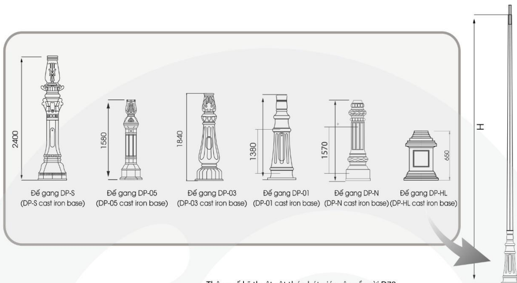
Thông số kỹ thuật cột thép bát giác côn cân rời D78
