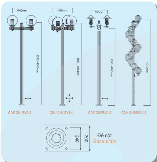
CỘT ĐÈN TRANG TRÍ THÂN NHÔM C04 | ALUMINUM BODY DECORATIVE LAMP POST C04
