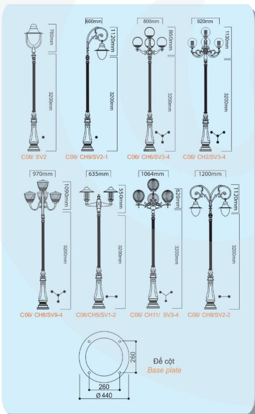
CỘT ĐÈN TRANG TRÍ ĐẾ GANG C06 | C06 DECORATIVE LAMP POST WITH CAST IRON BASE
