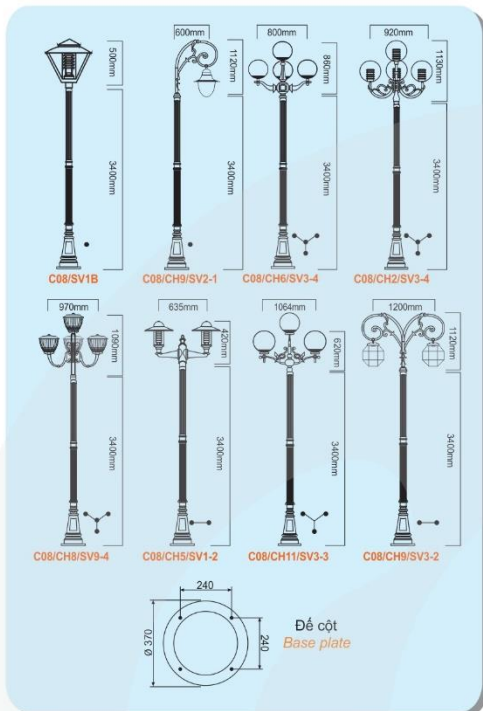
CỘT ĐÈN TRANG TRÍ ĐẾ GANG C08 | C08 DECORATIVE LAMP POST WITH CAST IRON BASE
