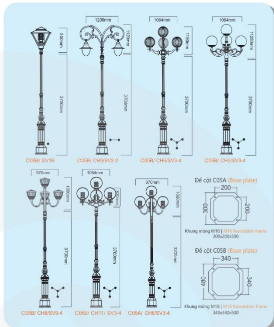
CỘT ĐÈN TRANG TRÍ ĐẾ GANG C05 | C05 DECORATIVE LAMP POST WITH CAST IRON BASE
