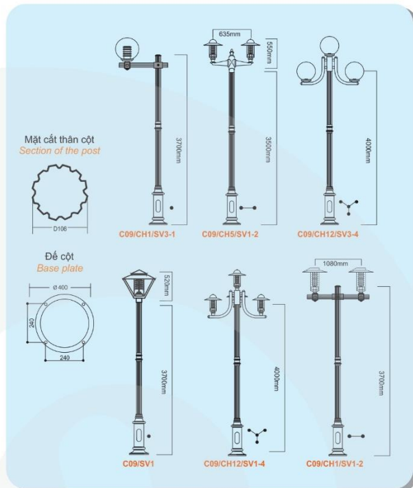
CỘT ĐÈN TRANG TRÍ ĐẾ NHÔM C09 | DECORATIVE LAMP POST WITH ALUMINUM BASE C09
