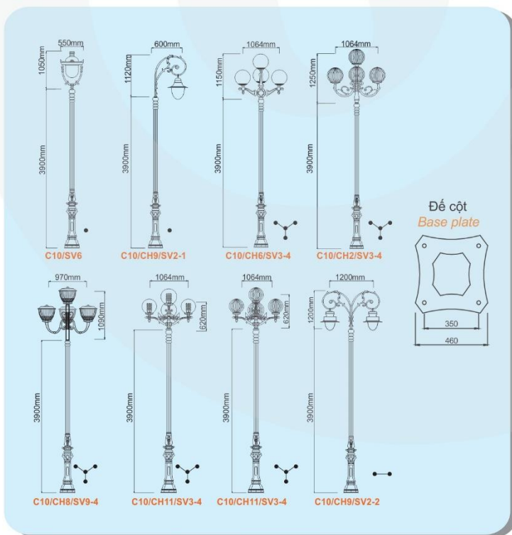
CỘT ĐÈN TRANG TRÍ ĐẾ GANG C10 | C10 DECORATIVE LAMP POST WITH CAST IRON BASE
