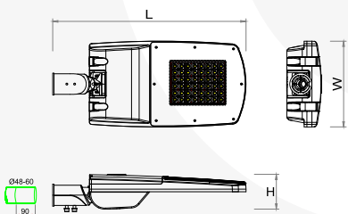
Bản vẽ hình chiếu (Dimensions)
